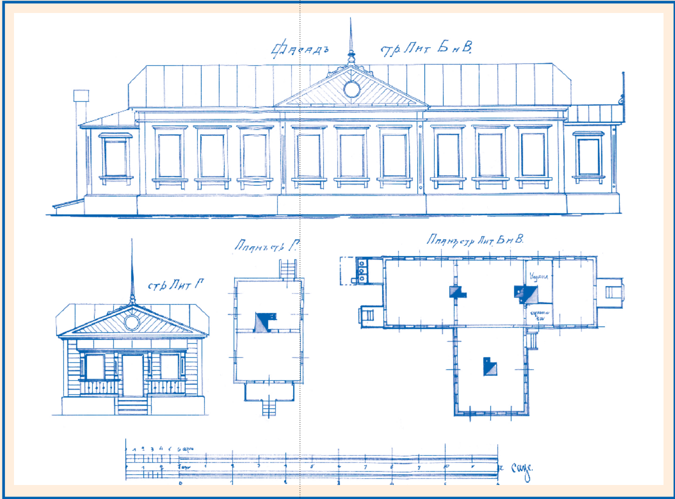
Фасады и планы строений на кирпичном заводе братьев Новиковых. 1914 год. Из фондов ЦИАМ.
